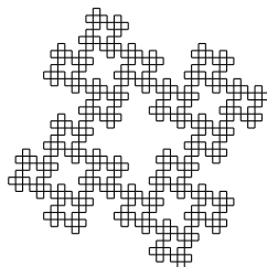
Abbildung 1: Ketten-Code-Anwendungen
