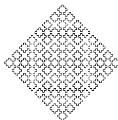
Abbildung 1: Ketten-Code-Anwendungen
